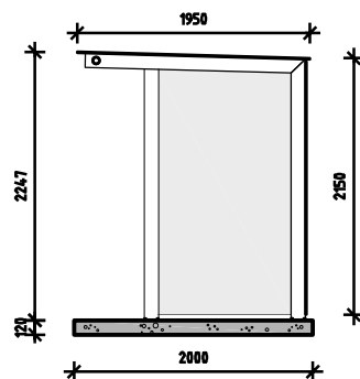
Dwarsdoorsnede
